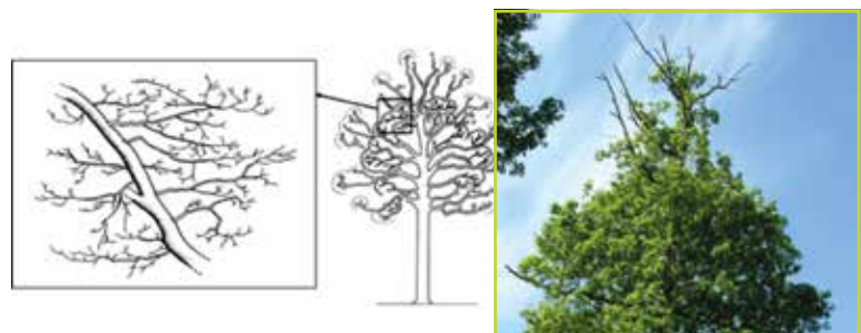
Figuur 7: links: morfologie van de hele boom (waterloten in vet) en detail van een tak met plagiotrope waterloten; rechts foto van een kroon van een zomereik met natuurlijke kroonreductie
