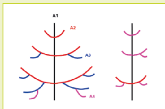
Figuur 12: schematische voorstelling van normale (links) en verarmde (rechts) vertwijging
