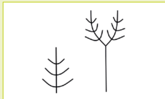
Figuur 11: schematische voorstelling van re-iteratie bij een jonge boom (rechts), herhaling van het basismodel (links)
