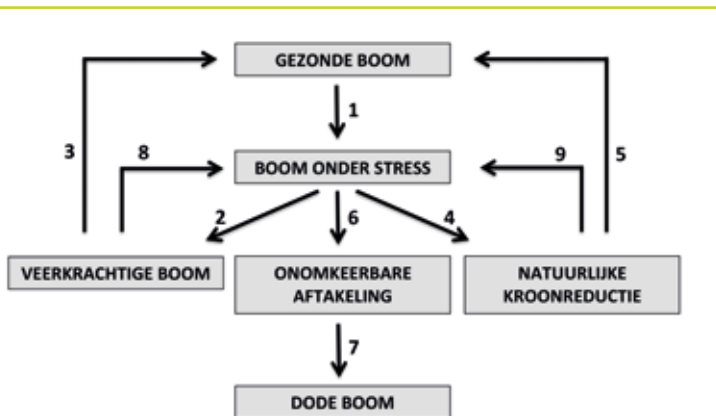
Figuur 1: de verschillende architecturale types en hun relaties
