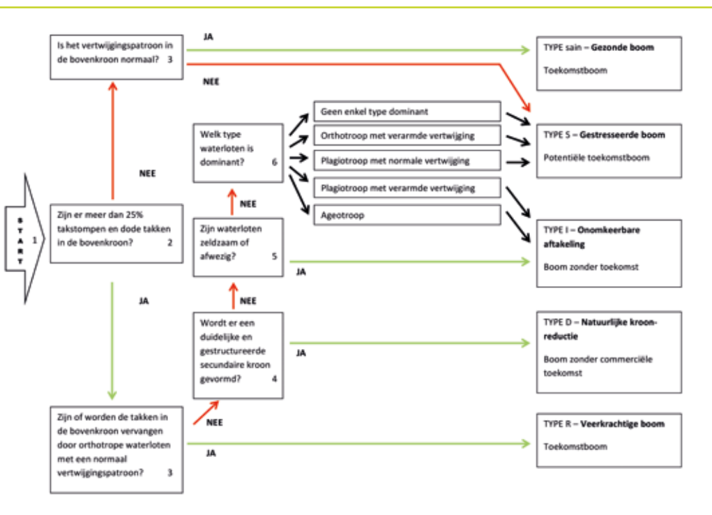
Figuur 3: Wintersleutel voor ARCHI-types bij zomereik. Cijfers verwijzen naar onderstaande tekst.
