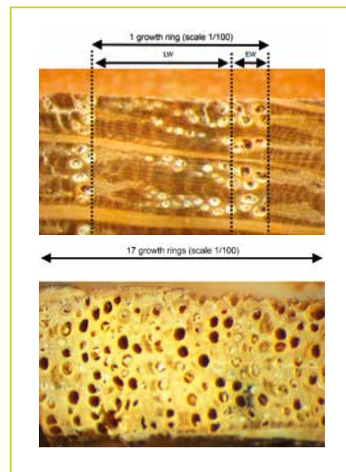
Figuur 4: boven: één jaarring van een eik van type R (veerkrachtig); onder: zeventien jaarringen van een eik van type I (onomkeerbare aftakeling). Beide foto's zijn op dezelfde schaal.
